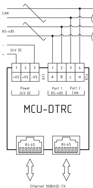
Схема подключения MCU-DTRC
