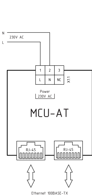
Схема подключения MCU-AT
