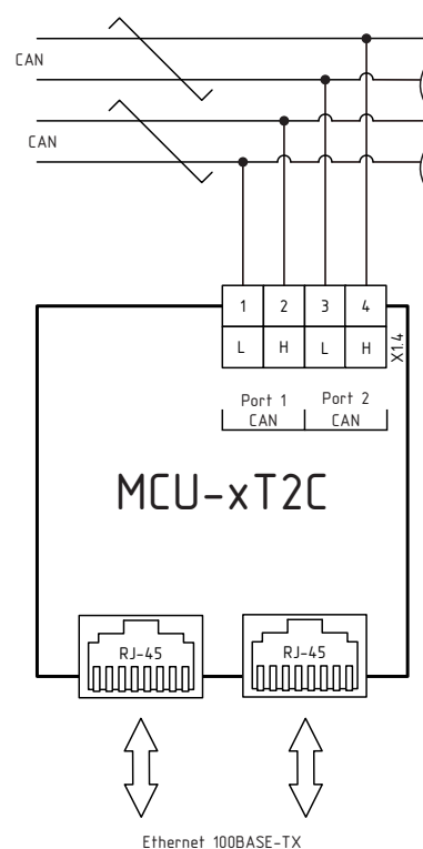
Схема подключения MCU-xT2C
